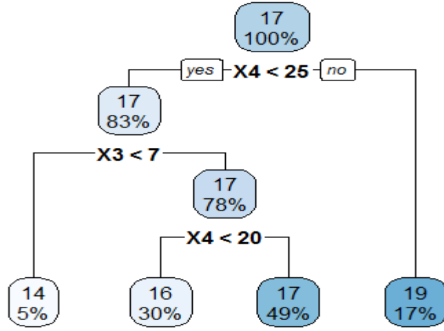
Şekil 4. % 7.5 Oranında Kayıp Veri İçeren Veri Seti için Regresyon Ağacı Diyagramı
