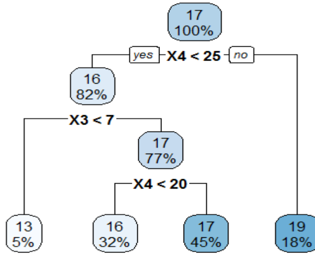
Şekil 1. Kayıp Veri İçermeyen Veri Seti için Regresyon Ağacı Diyagramı
