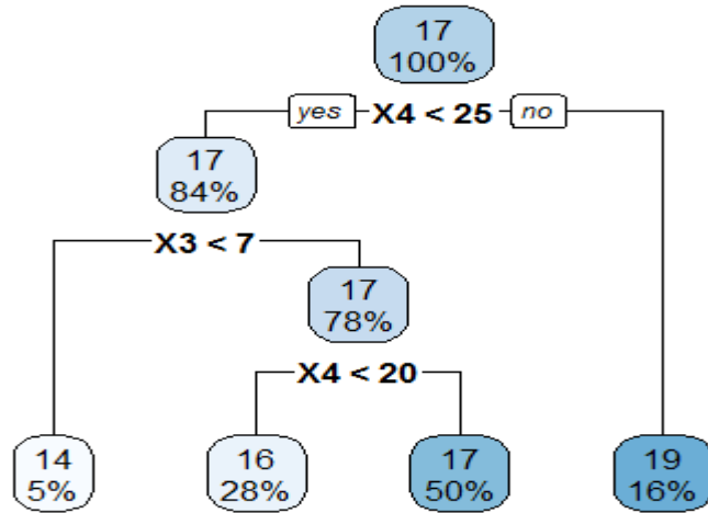
Şekil 5. % 10 Oranında Kayıp Veri İçeren Veri Seti için Regresyon Ağacı Diyagramı
