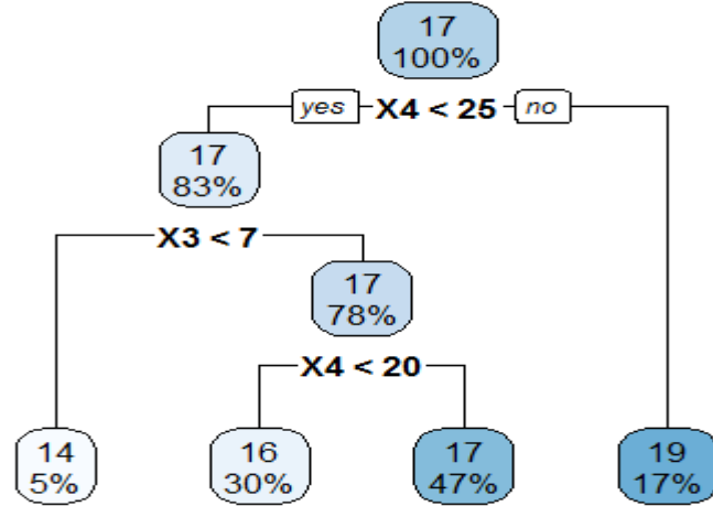
Şekil 3. % 5 Oranında Kayıp Veri İçeren Veri Seti için Regresyon Ağacı Diyagramı
