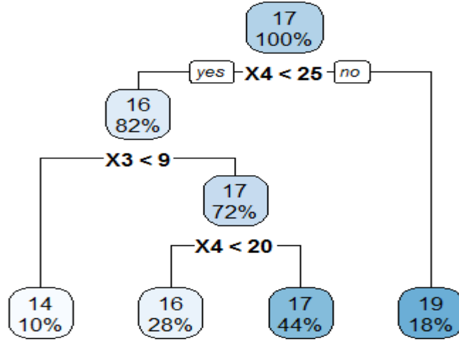
Şekil 2. % 2.5 Oranında Kayıp Veri İçeren Veri Seti için Regresyon Ağacı Diyagramı
