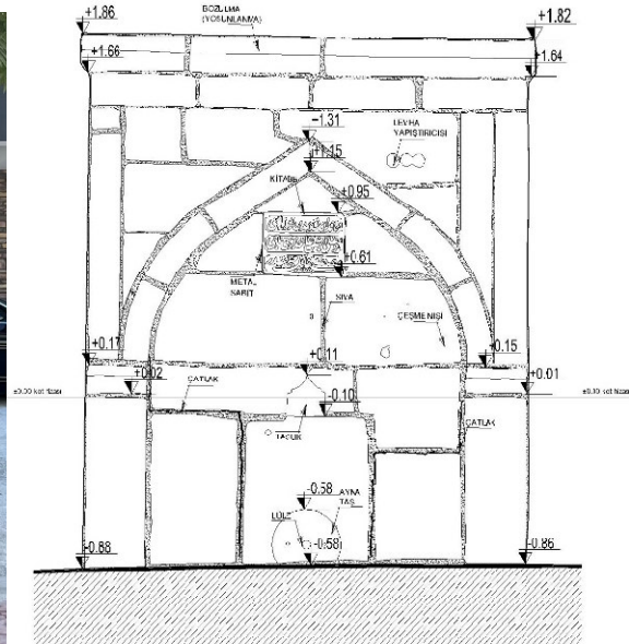
Şekil 10. Çeşmenin kuzeybatı (ön) cephesi görseli (H. Sevde Demir arşivi) Şekil 11. Çeşmenin kuzeybatı (ön) cephesinin mimari çizimi (Kübra Söğütlü-H. Sevde Demir)
