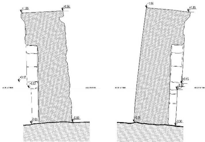
Şekil 13. Çeşmenin yan cephelerinin mimari çizimi (H. Kübra Söğütlü- H. Sevde Demir)
